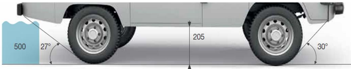
UAZ FURGÓN 4x4: 5 ASIENTOS CON VIDRIOS - 2 ASIENTOS SIN VIDRIOS
